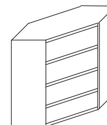
skř. rohová (H15) 75x75/90/30
