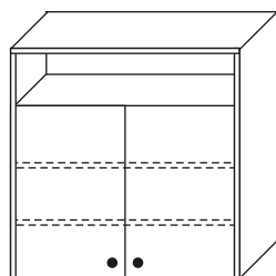
skř. dvoudveřová (H13) 90/90/31,8
